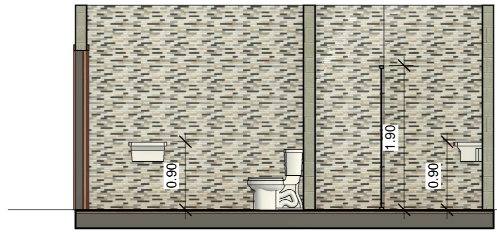
2 Corte 1 1 : 50
