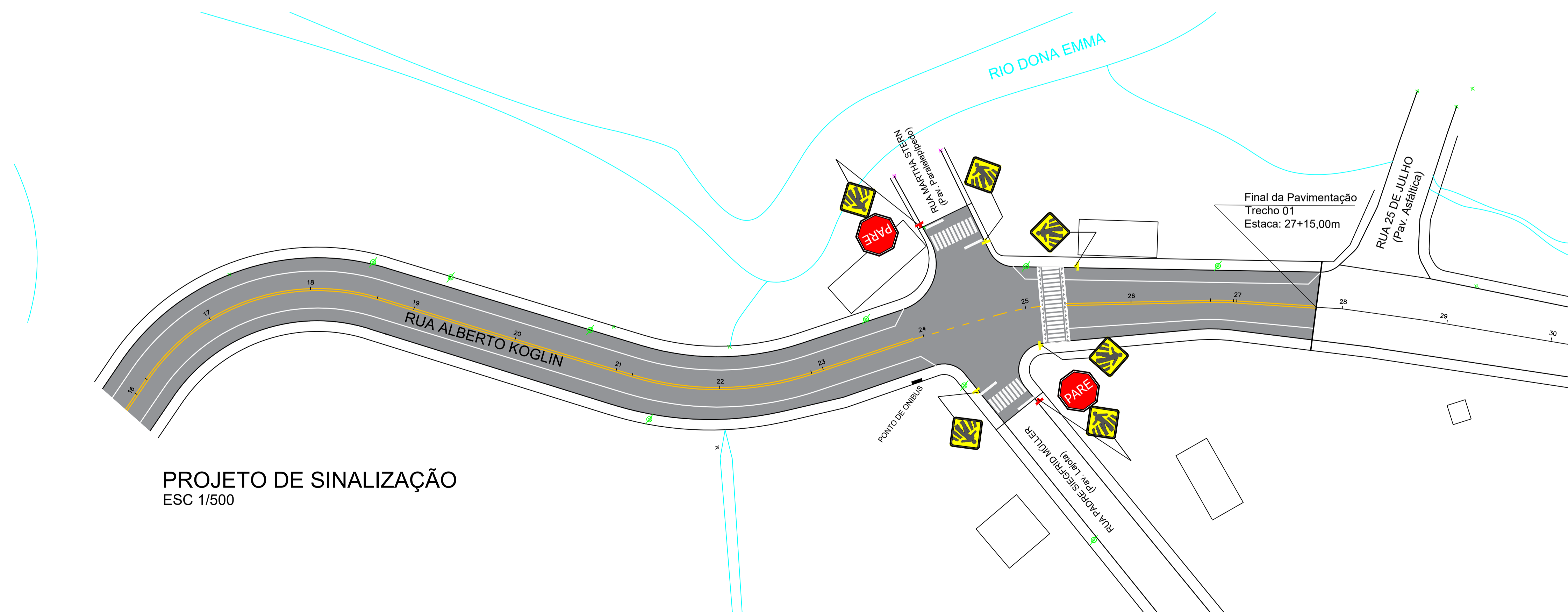
PROJETO DE SINALIZAÇÃO ESC 1/500
