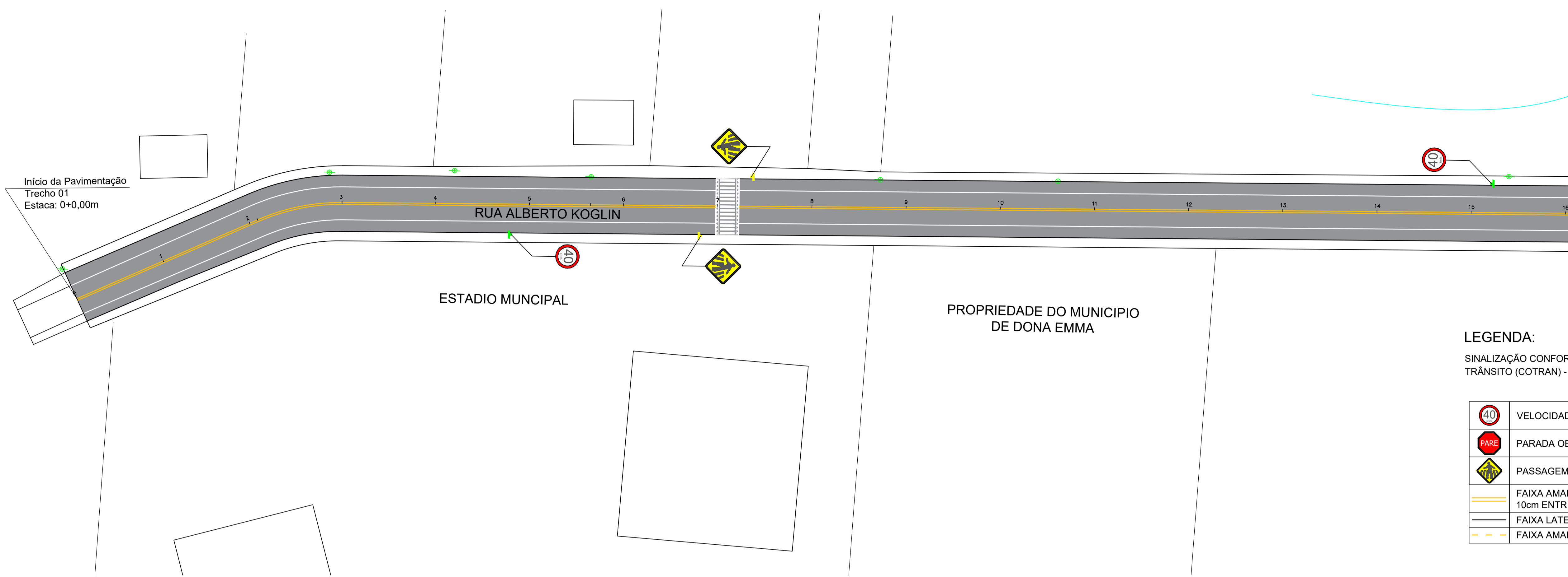
PROJETO DE SINALIZAÇÃO ESC 1/500
