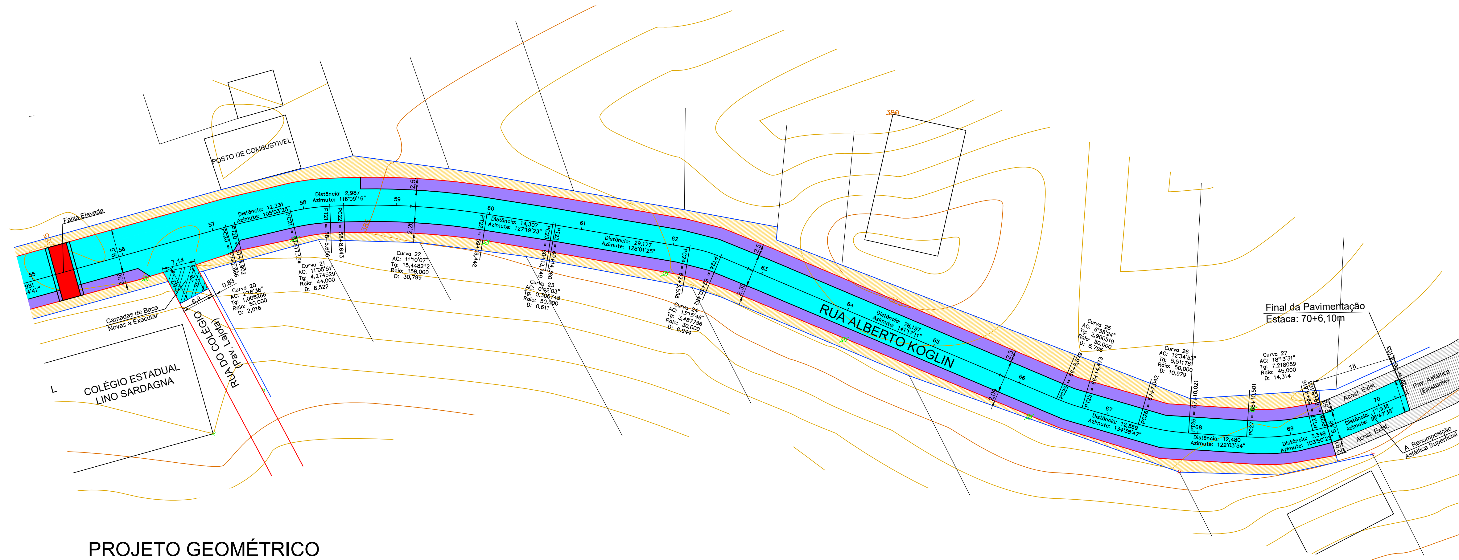
PROJETO GEOMÉTRICO ESC 1/500
